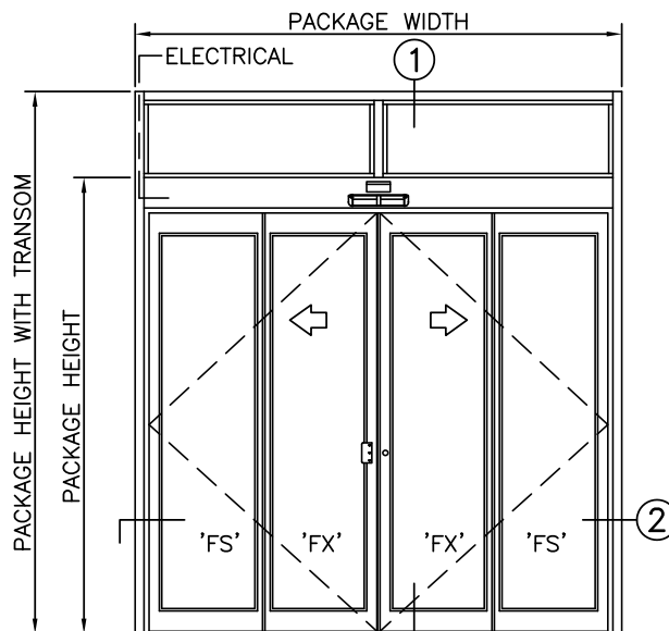
ELEVATION
