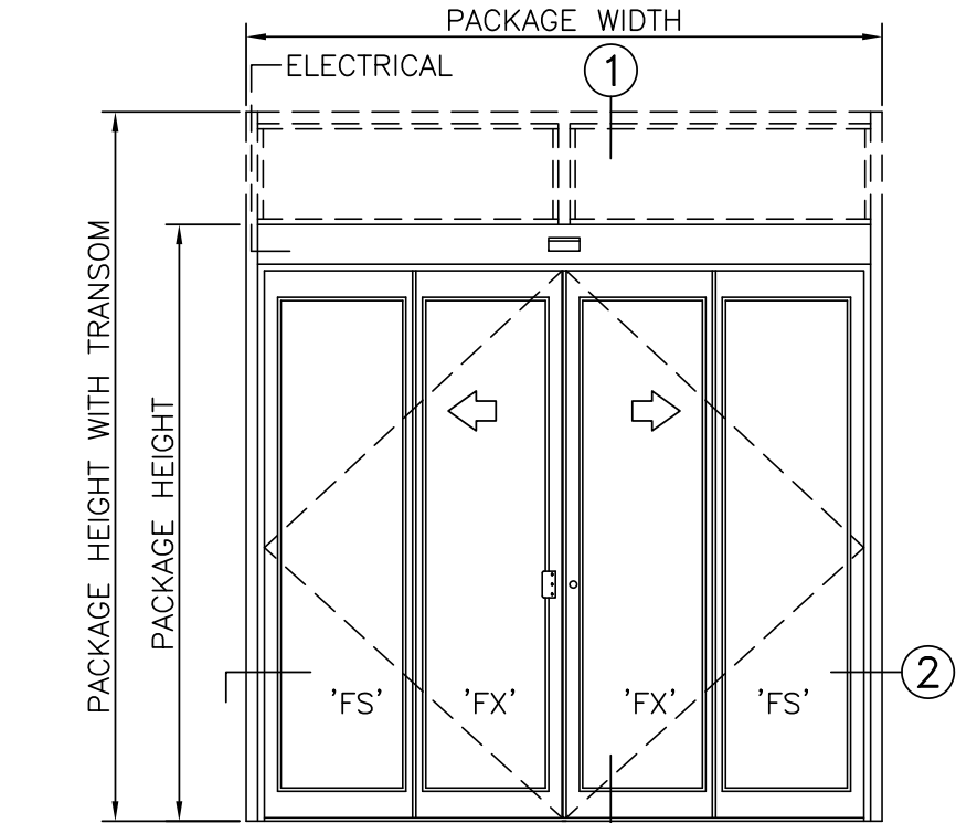
ELEVATION VIEW SCALE: 3/8" = 1'-0"
