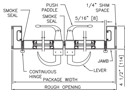
HORIZONTAL SECTION (PAIR)
