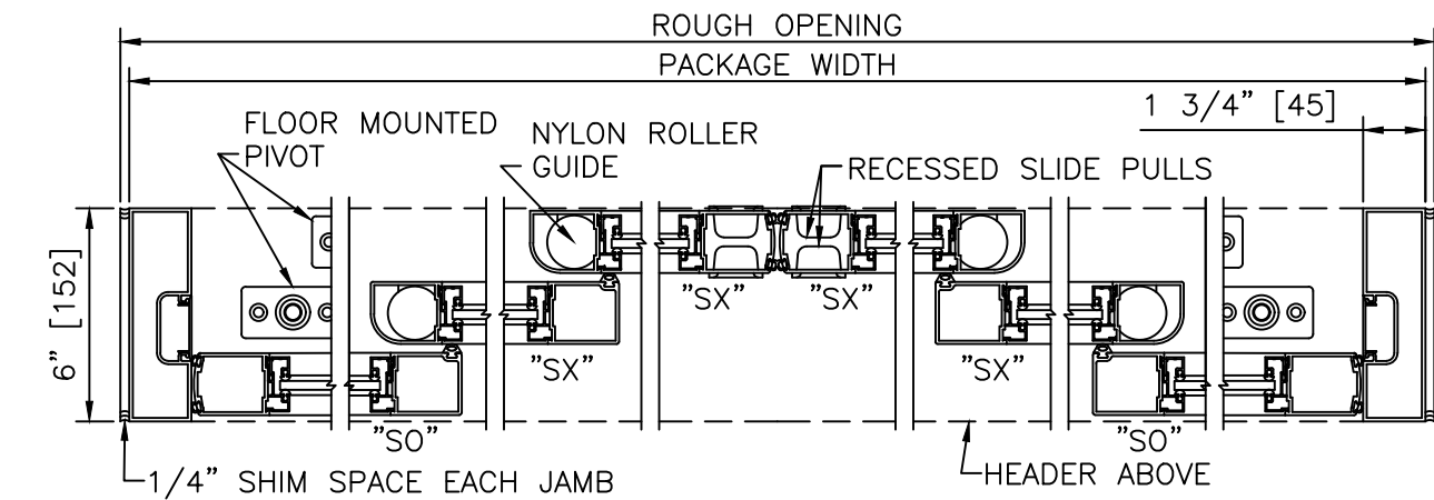
2 HORIZONTAL SECTION SCALE: 2" = 1'-0"
