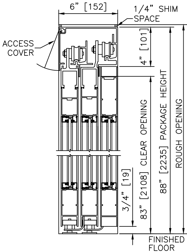
1 VERTICAL SECTION SCALE: 2" = 1'-0"
